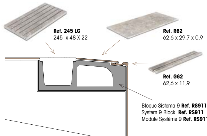
Piscina desbordante: Nuevo sistema Horyzon Deck level Pool: New Horyzon system Systèmes à débordement: Nouveaux système Horyzon
